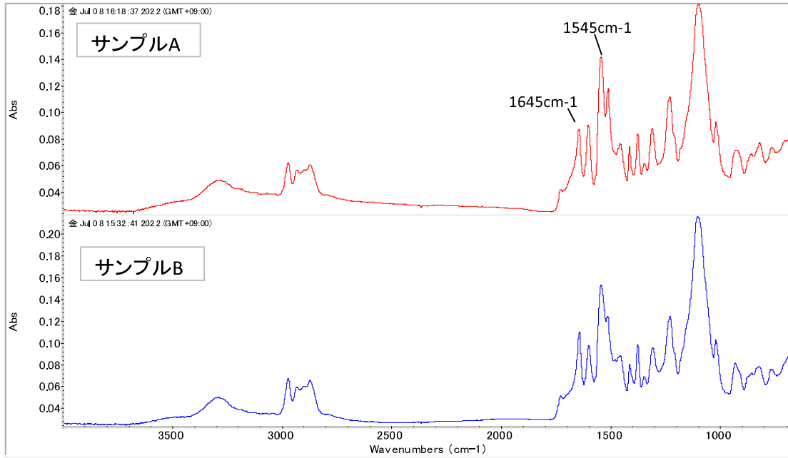
図2 IRスペクトル比較
