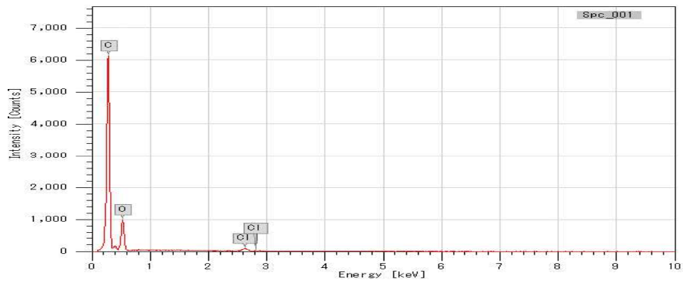
図1 定性チャート
